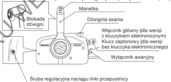
MANETKA ZDALNEGO STEROWANIA
